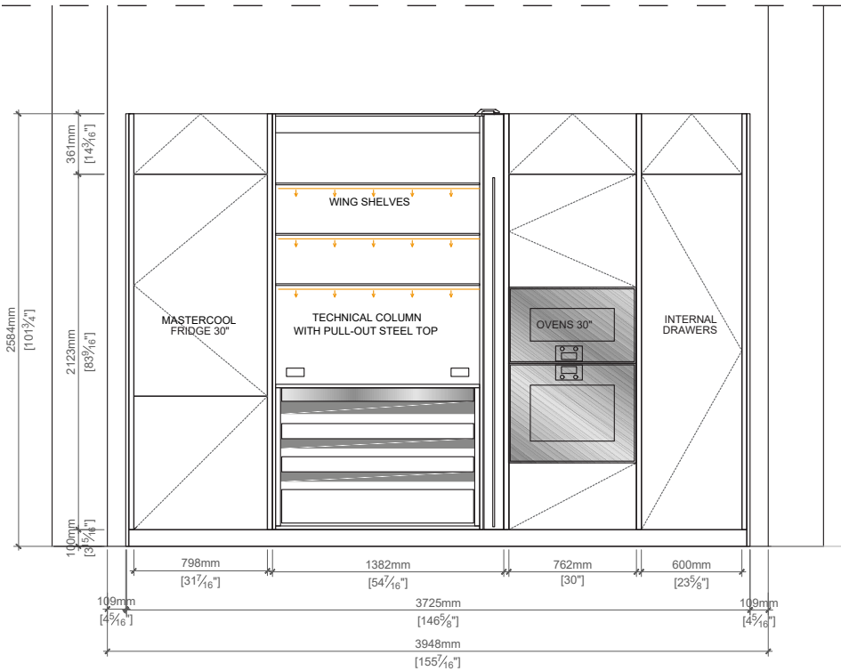
Elevation A
